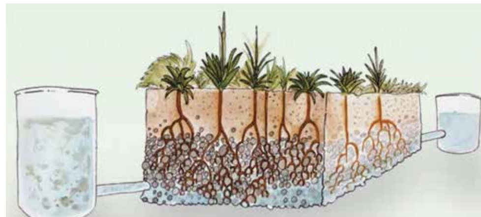
Fig. 1 Il meccanismo della fitodepurazione. Le acque reflue eccessivamente ricche di sostanze organiche vengono fatte scorrere attraverso un substrato ghiaioso ricoperto da essenze vegetali adatte. Durante il passaggio, i meccanismi chimici e fisici innescati dalla presenza di minerali e della flora e della fauna presenti nel sistema, favoriscono la riduzione del carico organico presente e la conseguente depurazione delle acque che vengono restituite all'ambiente.
